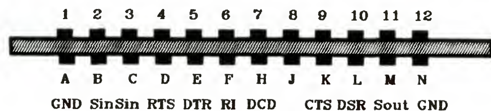
Port szeregowy — C-64, C-128, PLUS/4
