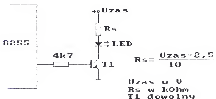
Rys. 3 Podłączenie LED
