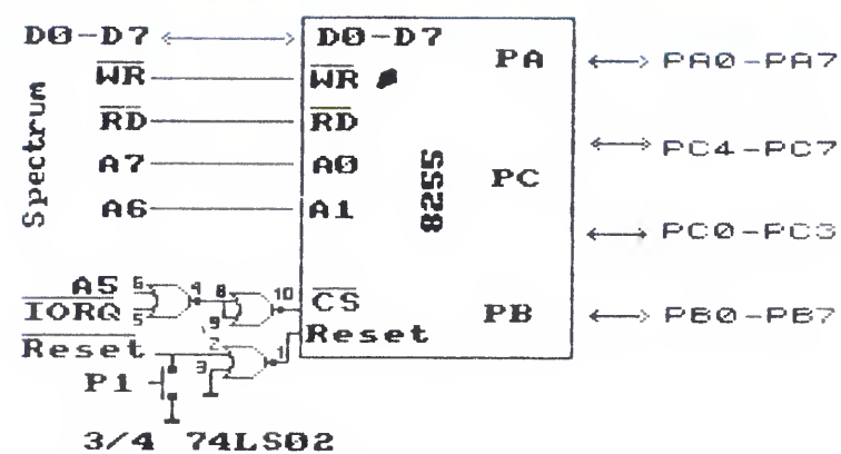
Rys. 1 Schemat interfejsu.
