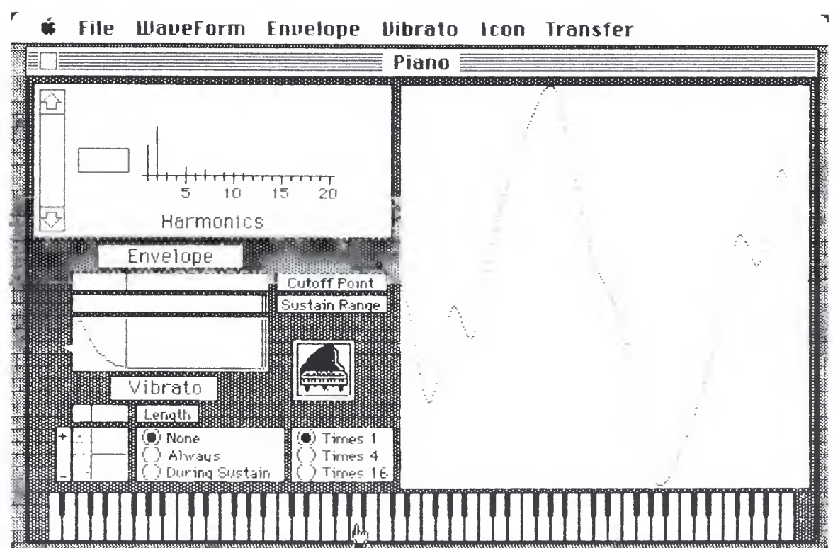
Rys. 3 Edytor instrumentów
