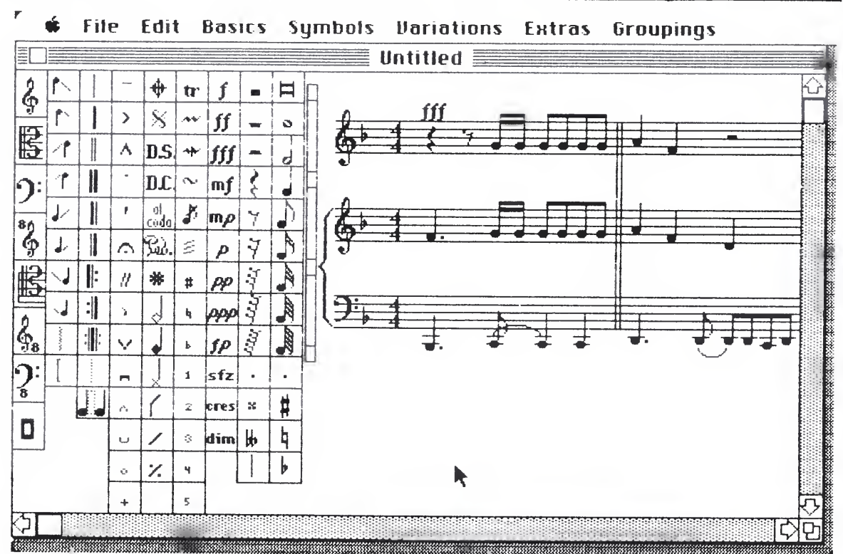
Rys. 1 Edytor
