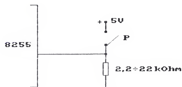
Rys.2 Podłączenie przełącznika.
