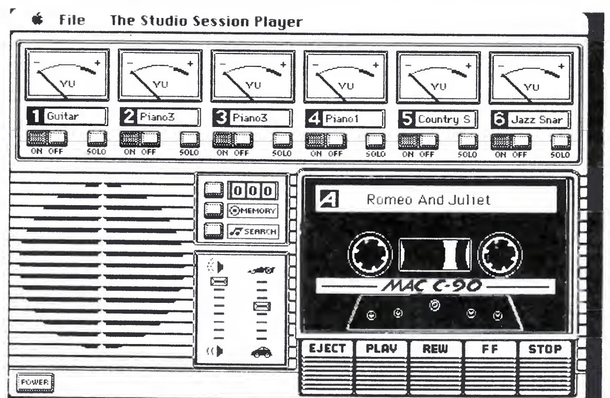
Rys. 2 Odtwarzacz
