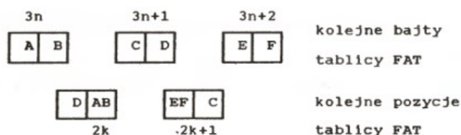
Rys. 3. Wyznaczanie dwóch kolejnych pozycji tablicy FAT na podstawie trzech kolejnych bajtów tej tablicy.
