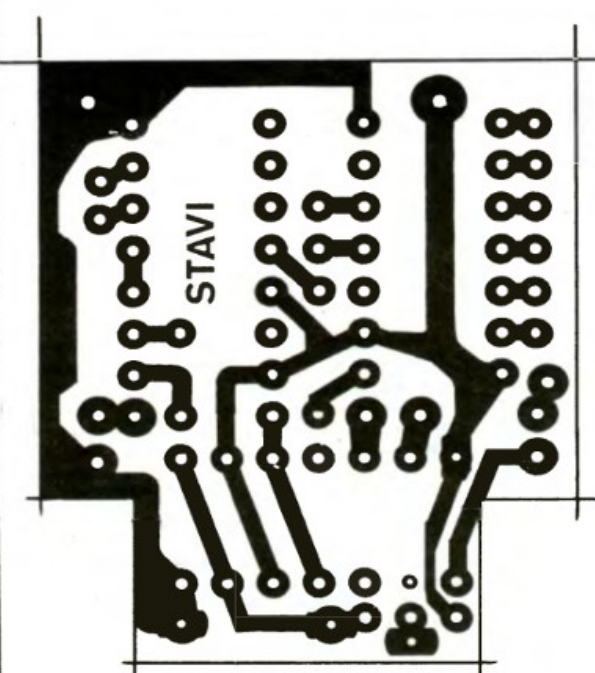
Rys. 2a Rysunek płytki drukowanej
