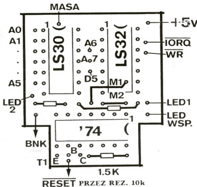
Rys. 2b Rozmieszczenie elementów i sygnałów
