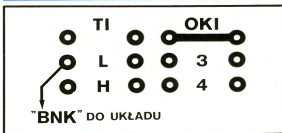
Rys. 3 Podłączenie sygnału BNK
