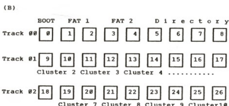
Rys. 2. Numeracja i opis sektorów dyskiety. (A) 2-stronna, 40 ścieżek, 9 sekt/ścieżkę (B) 1-stronna, 40 ścieżek, 9 sekt/ścieżkę
