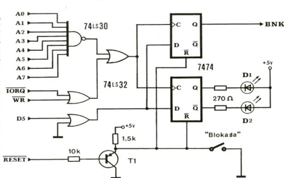
Rys. 1 Schemat układu przełączania banków
