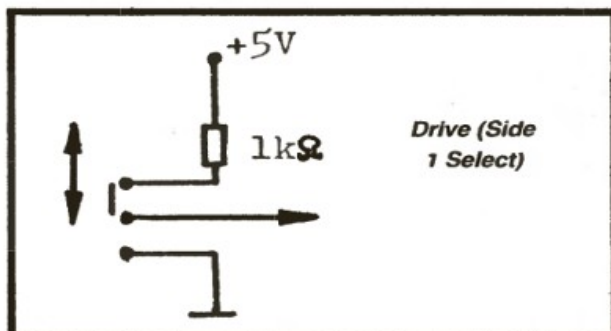
Wybór strony dla drive'u 2x40 TRACK
