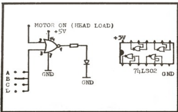
Podłączenie diody
