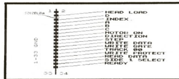
Rys. 2 Złącze z sygnałami
