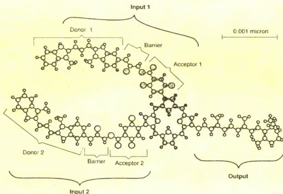
Rys. 1. Molekularna bramka typu NAND sterowana światłem laserowym. Ma ona rozmiar rzędu 4 nm i jest 10000 razy szybsza od jej krzemowego odpowiednika. Składa się z dwóch wejść (Input 1, Input 2) i jednego wyjścia (Output). Łańcuch odpowiadający każdemu z wejść zawiera trzy części: obszar donora, barierę i obszar akceptora.
