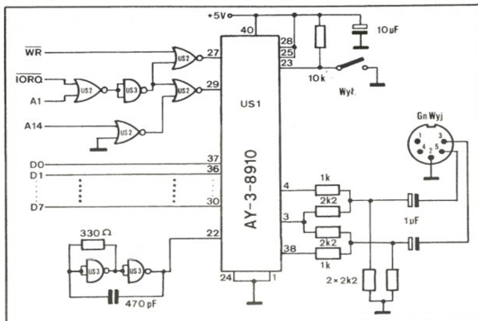
Rys. 1 Schemat ideowy przystawki
