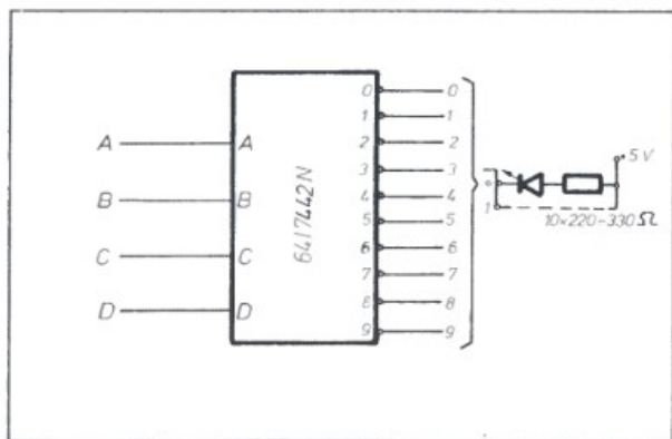
Rys. 2 — przy zastosowaniu układu UCY 7442 (dekoder 1 z 10) możliwe jest sekwencyjne sterowanie 10 diodami. Wykorzystując program przedstawiony w pierwszej części artykułu uzyskamy efekt przesuwającego się punktu świetlnego. Oczywiście zamiast diod można zastosować elektroniczne włączniki uruchamiające dowolne urządzenia. W następnej części artykułu postaram się przedstawić możliwości sterowania różnymi urządzeniami w zależności od stanu określonych czujników.
