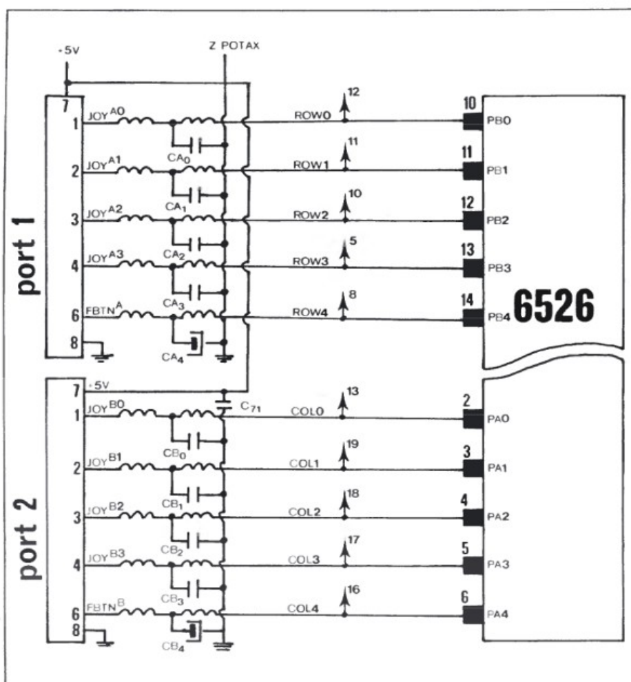
Rys. 1. Połączenie portów drążków z układem CIA — Commodore 64. Strzałki wskazują połączenie linii ze złączem klawiatury.
