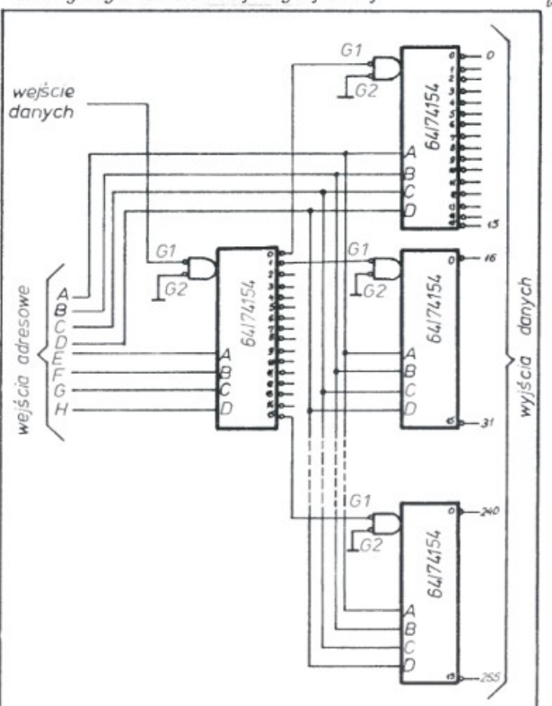
Rys. 5 — przedstawiony schemat jest propozycją wykorzystania portów joysticków do sterowania 256 urządzeniami. Bliższe informacje na temat tego układu, układów przedstawionych wcześniej oraz innych ciekawych rozwiązań można znaleźć w książce W. Sasala pt. „Układy scalone serii UCA64/UCY74, parametry i zastosowania”, WKiŁ, 1985.
