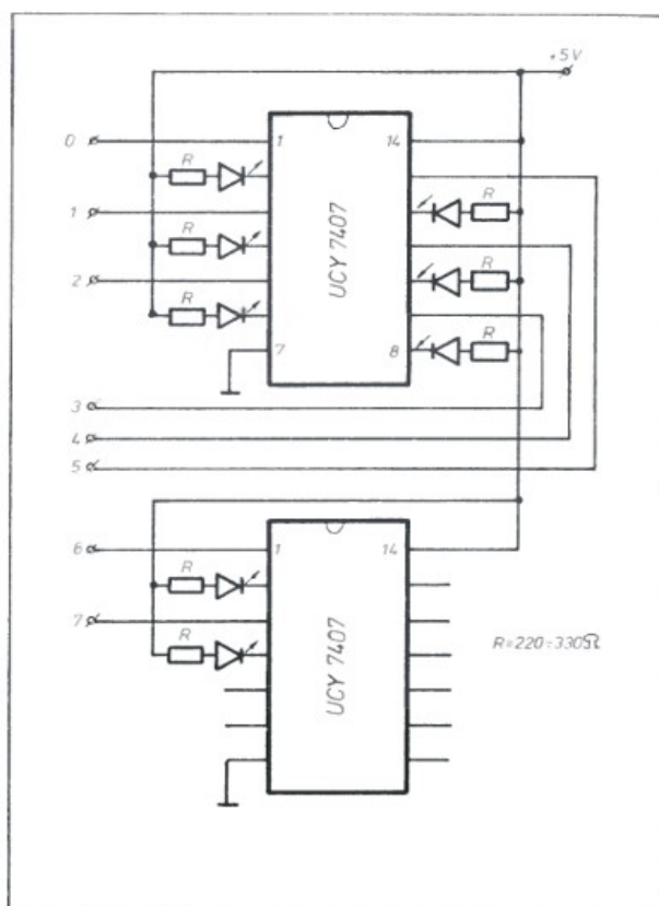
Rys. 1 — przedstawiono na nim schemat układu umożliwiającego uzyskanie dużej jasności świecenia diod. Wartości rezystorów R należy dobrać tak, aby uzyskać odpowiednią jasność, ale nie przekroczyć dopuszczalnej wartości prądu płynącego przez diodę. Uwaga ta odnosi się do wszystkich przedstawionych układów.
