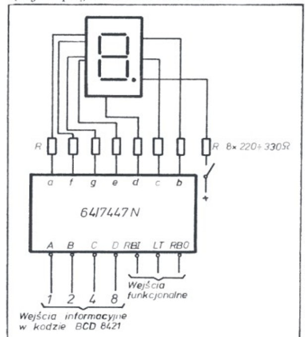
Rys. 4 — jest to najpopularniejszy dekoderny kod binarnego na kod wskaźnika siedmiosegmentowego. Umożliwia on wzrokową obserwację aktualnej wartości pojawiającej się w wybranym porcie joysticków. Można do każdego portu dołączyć taki układ i stworzyć prosty program na przykład do podglądania zawartości określonych rejestrów, stoper czy programowalny zegar do ciemni fotograficznej.
