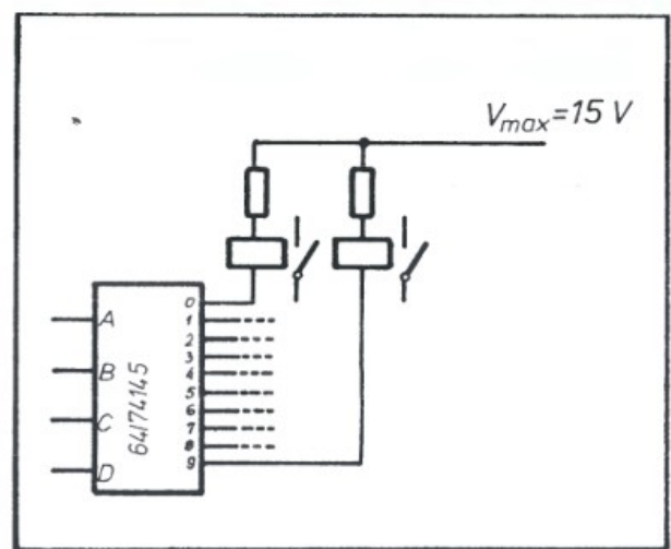
Rys. 3 — jest to w zasadzie taki sam układ jak opisany wyżej. Różnica polega jedynie na zastosowaniu dekodera z obwodem otwartego kolektora w stopniu wyjściowym. Dzięki temu możliwe jest dołączenie przełączników na inne napięcie niż 5V, jednak nie wyższe niż 15V. Do styków przełączników można dołączyć na przykład żarówki sieciowe.
