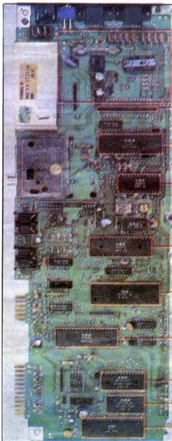
Rys 2. PŁYTA GŁÓWNA NOWEGO C-64
