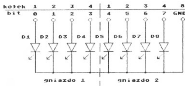
Rys. 2. Przyłączenie diod do gniazd joysticków (D1-D8 — dowolne diody elektroluminescencyjne typu CQYP).
