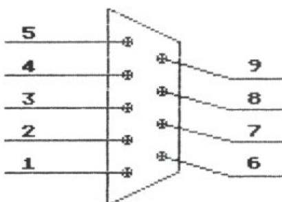
Rys. 1. Połączenie PORTA z gniazdami joysticków.
