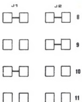
Rys. 3. Kombinacje połączeń złączy J1 i J2 i odpowiadające im numery urządzenia.
