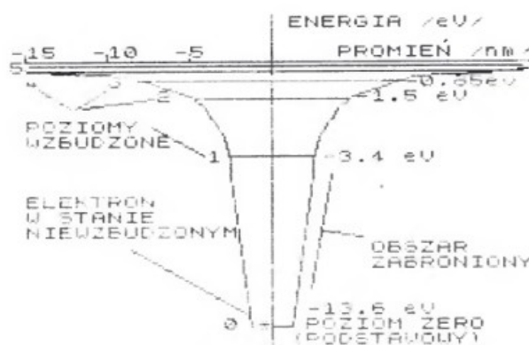
Rys. 1. Dół energetyczny elektronu w atomie wodoru.
