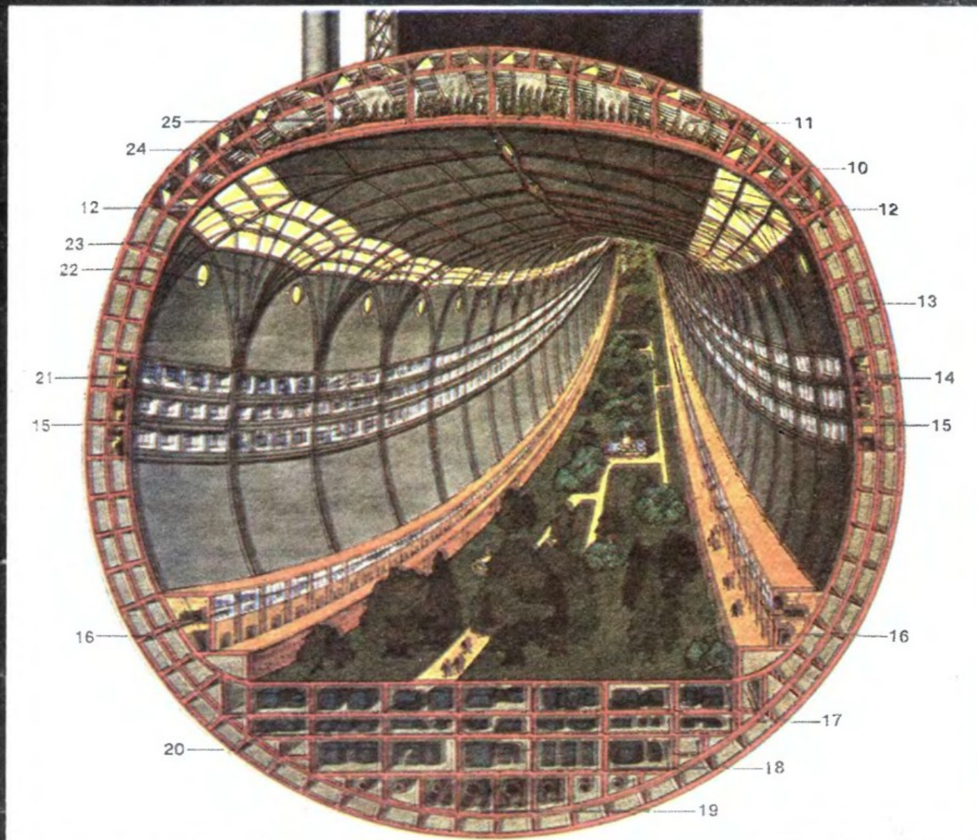
Przekrój poprzeczny kosmicznego miasta typu toroidalnego. 10. Lustro oświetlające okna głównej przestrzeni życiowej miasta. 11. Lustro oświetlające strefę rolniczą. 12. Okna głównej przestrzeni życiowej miasta. 13. Bloki konstrukcyjne toroidu. 14. Aparatura w wewnętrznych sekcjach ścian. 15. Balkony. 16. Główna strefa mieszkalna miasta — z kawiarniami i sklepami na parterze. 17. Schrony awaryjne. 18. Strefa przemysłowa. 19. Podstawowe rurociągi i kable systemu zasilania i łączności. 20. Magazyny. 21. Zaplecze systemu sterowania. 22. Sztuczne oświetlenie. 23. Konstrukcje szkieletu wewnętrznego. 24. Dach (znajduje się w odległości 113 metrów od „ziemi”). 25. Strefa rolnicza.
