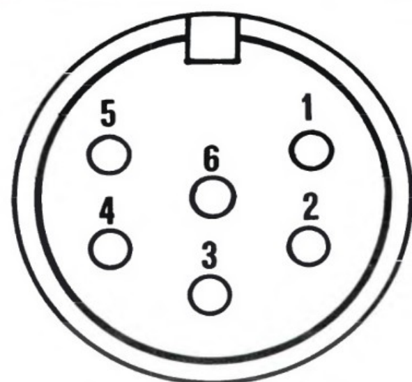
RYSUNEK 2 — Schemat wyprowadzeń portu szeregowego (SERIAL BUS) — widok z przodu
