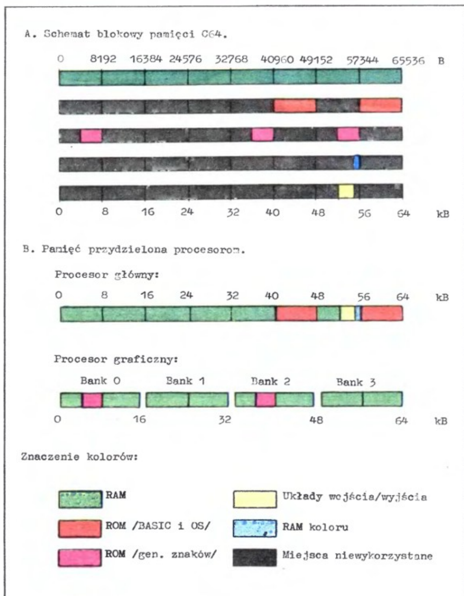
Rys.1 Mapa pamięci C64
