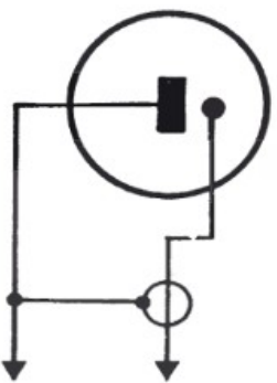
Rys. 2 Wtyk głośnikowy
