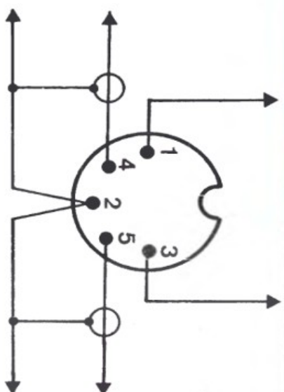
Rys. 3 Wtyk magnetofonowy komputera
