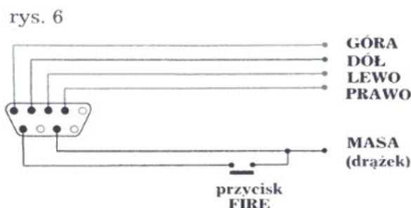
Widok wtyczki od strony połączeń. Przewody należy podłączyć do odpowiednich styków
