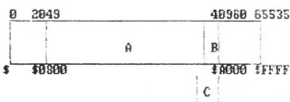
Rys. 2 A — obszar pamięci zajmowany przez program B — obszar pamięci pozostawiony dla zmiennych łańcuchowych C — obszar konieczny do wpisania tytułu.
