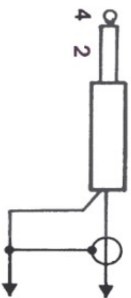
Rys. 1 Wtyk słuchawkowy
