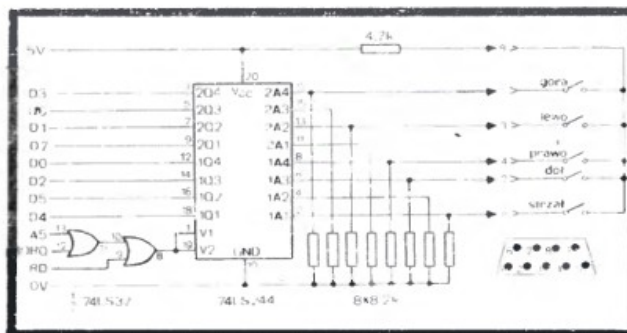
Rys.1. Schemat ideowy interfejsu i sposób podłączenia manipulatora.
