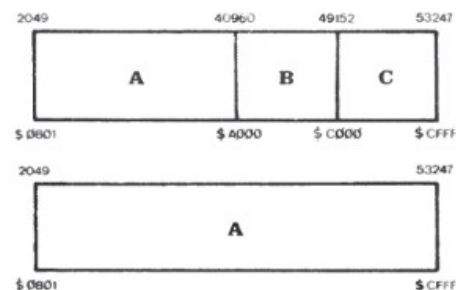
Rys.1. Konfiguracja pamięci przed wyłączeniem interpretera BASIC (a) oraz po jego wyłączeniu (b) A — Pamięć RAM dostępna dla użytkownika B — Obszar pamięci „maskowany” przez interpreter C — Dodatkowe 4 kb pamięci RAM nieadresowanej przez BASIC
