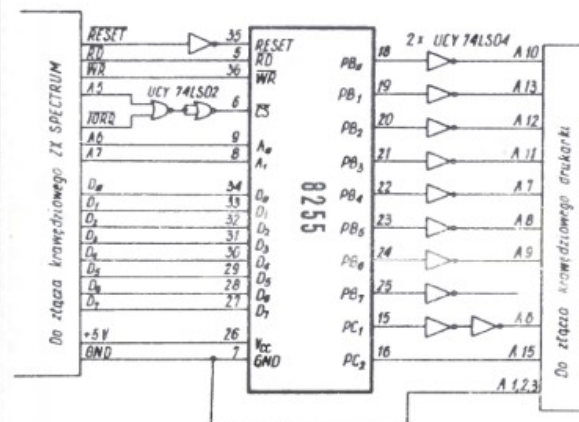
Rys. 1 Schemat ideowy interface'u
