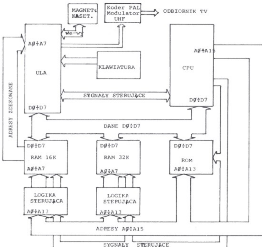
RYS. 1: Schemat blokowy ZX Spectrum 48K
