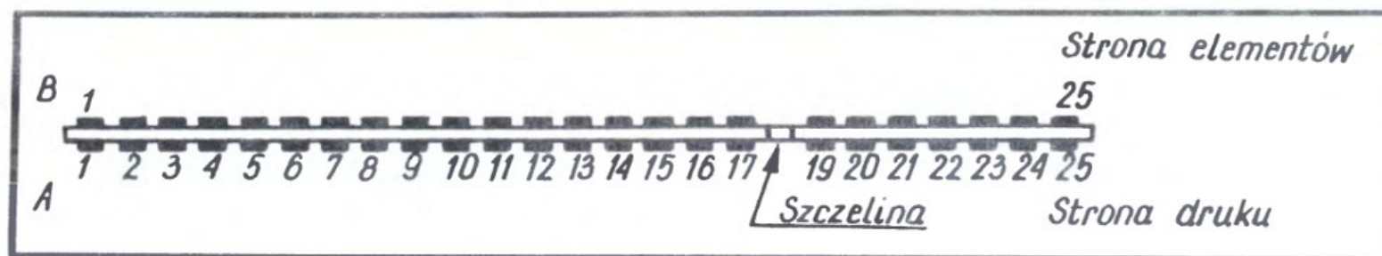
Schemat złącza krawędziowego drukarki DZM-180
