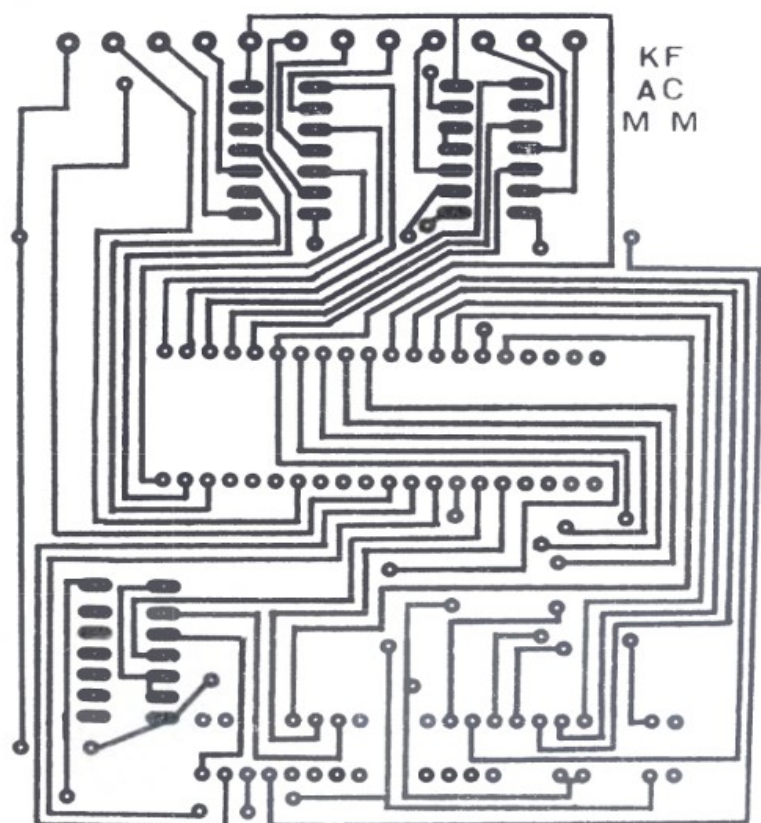
Rys. 2 Płytki drukowanej interfejsu skala 1:1
