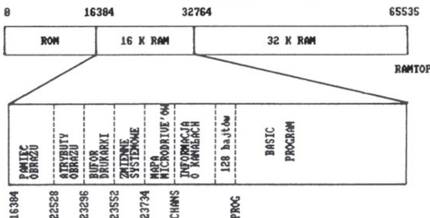
RYS. 2: Mapa pamięci
