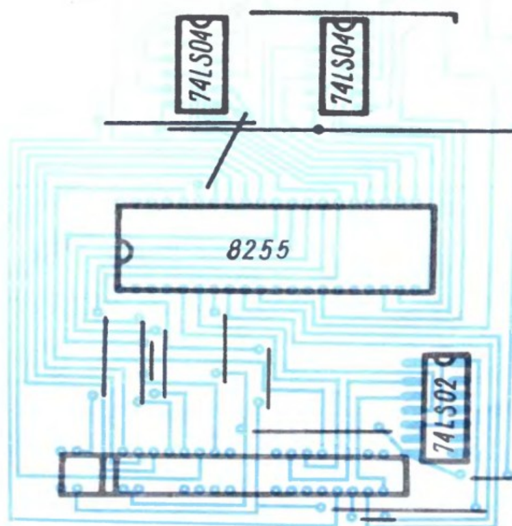
Rys. 3 Schemat montażowy, widok od strony elementów
