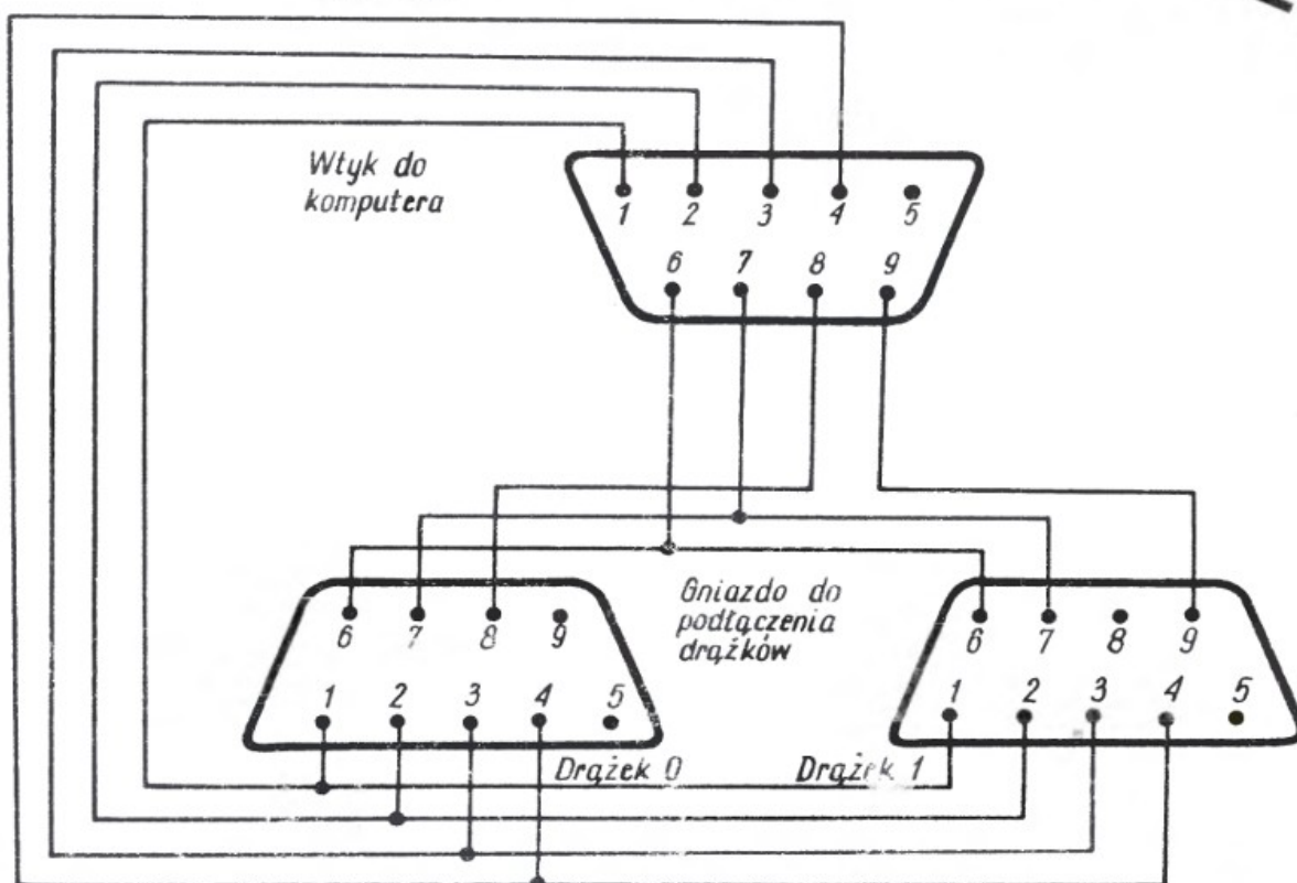
Rys.1. Schemat podłączenia dwóch drążków sterowych do mikrokomputera Amstrad-Schneider (widok gniazd i wtyczki od strony połączeń lutowniczych).
