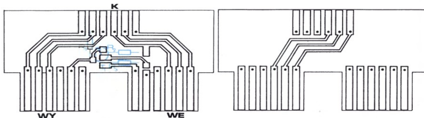
Rys. 2a i b. Ustawienie elementów na płytce
