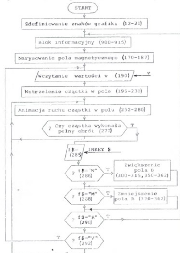
Rys. 2 Schemat blokowy programu.
