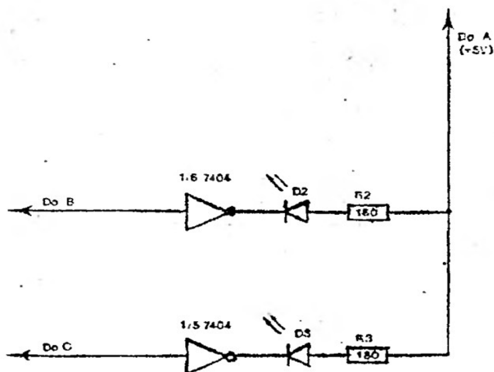
Rys. 3. Schemat ideowy sygnalizatora
