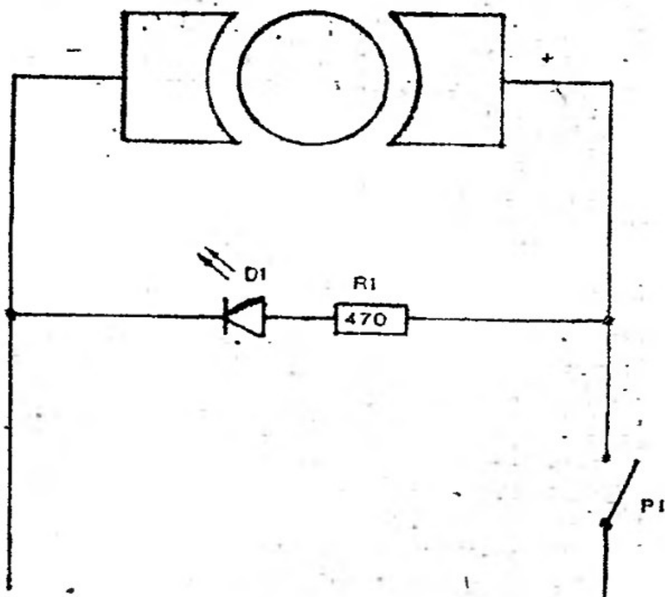
Rys. 4. Schemat podłączenia diody sygnalizującej pracę silnika
