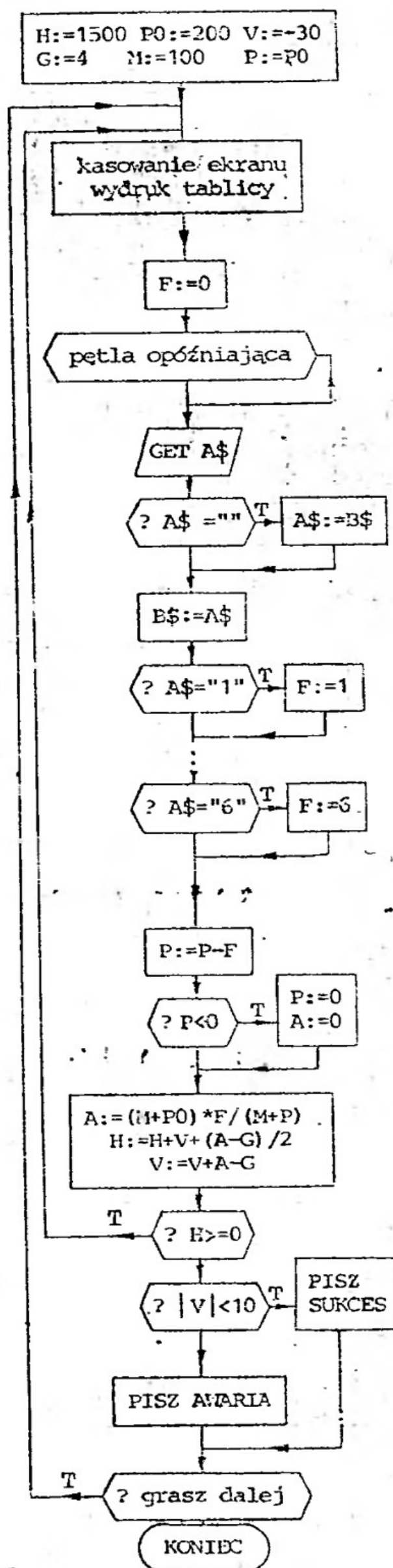
Schemat blokowy algorytmu
