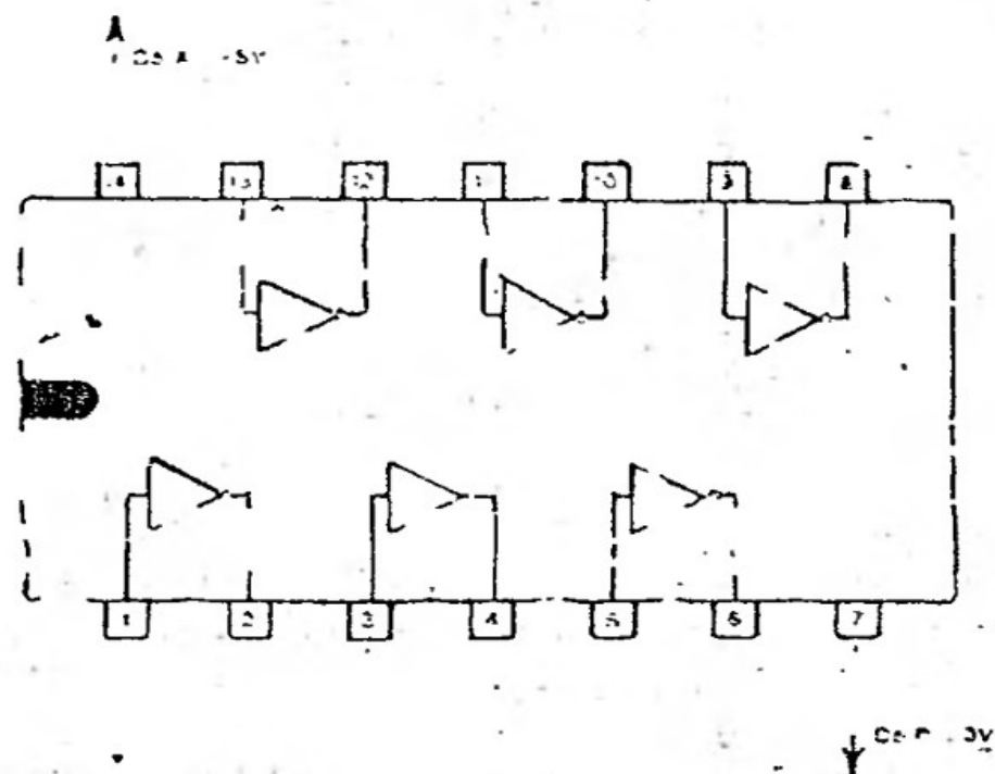
Rys. 1. Schemat wyprowadzeń układu UCY 7404 (widok z góry)
