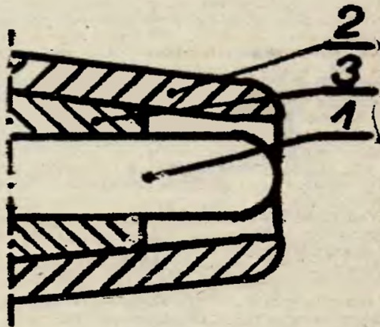
Rys. 5. Sposób zamocowania fototranzystora. 1 — fototranzystor, 2 — obudowa, 3 — podkładka gumowa.
