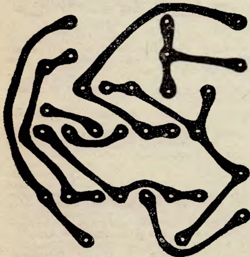
Rys. 3. Płytkę drukowaną — widok od strony miedzi (podz. 2:1).
