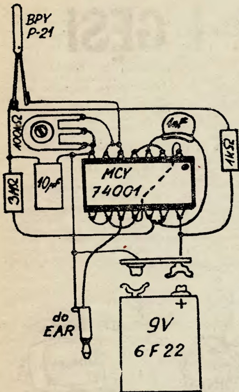
Rys. 2. Rysunek poglądowy, przedstawiający sposób montażu bezpośrednio do podstawki układu scalonego.
