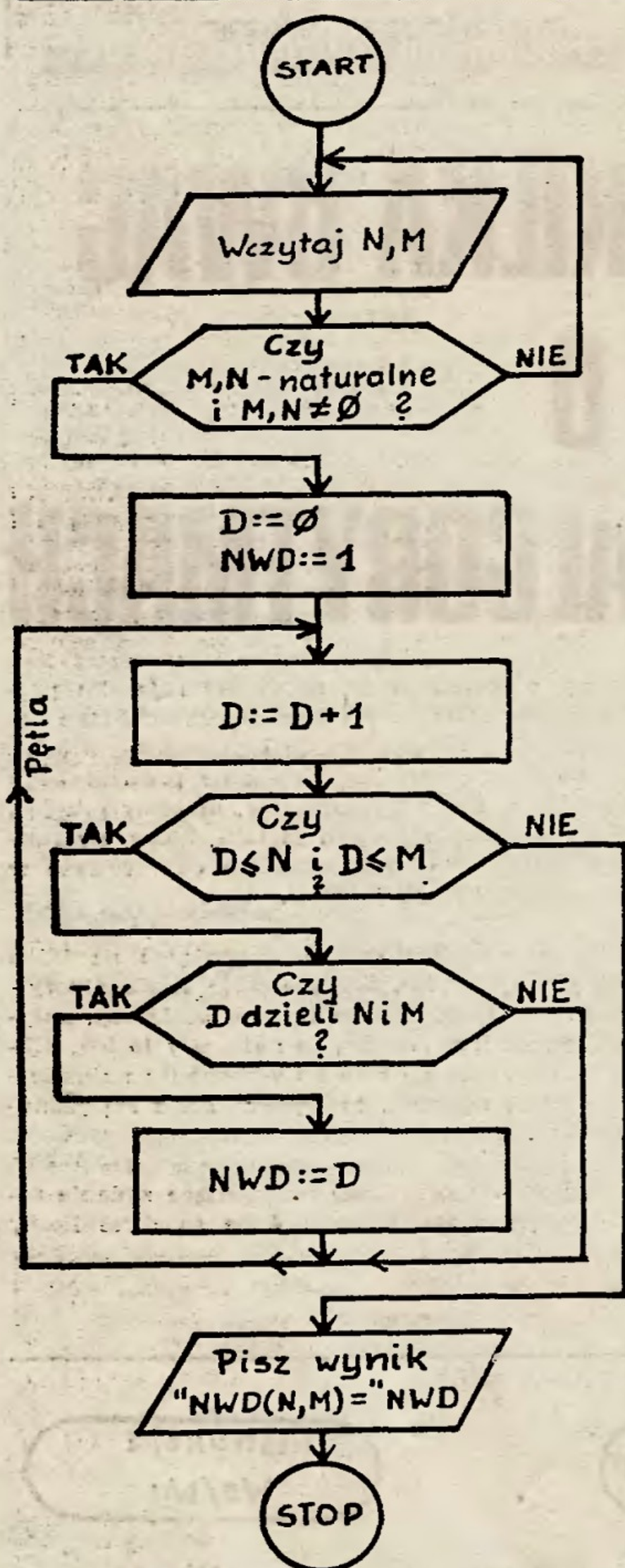
Rys. 2. Schemat blokowy algorytmu „siłowego” znajdowania NWD dwóch liczb naturalnych
