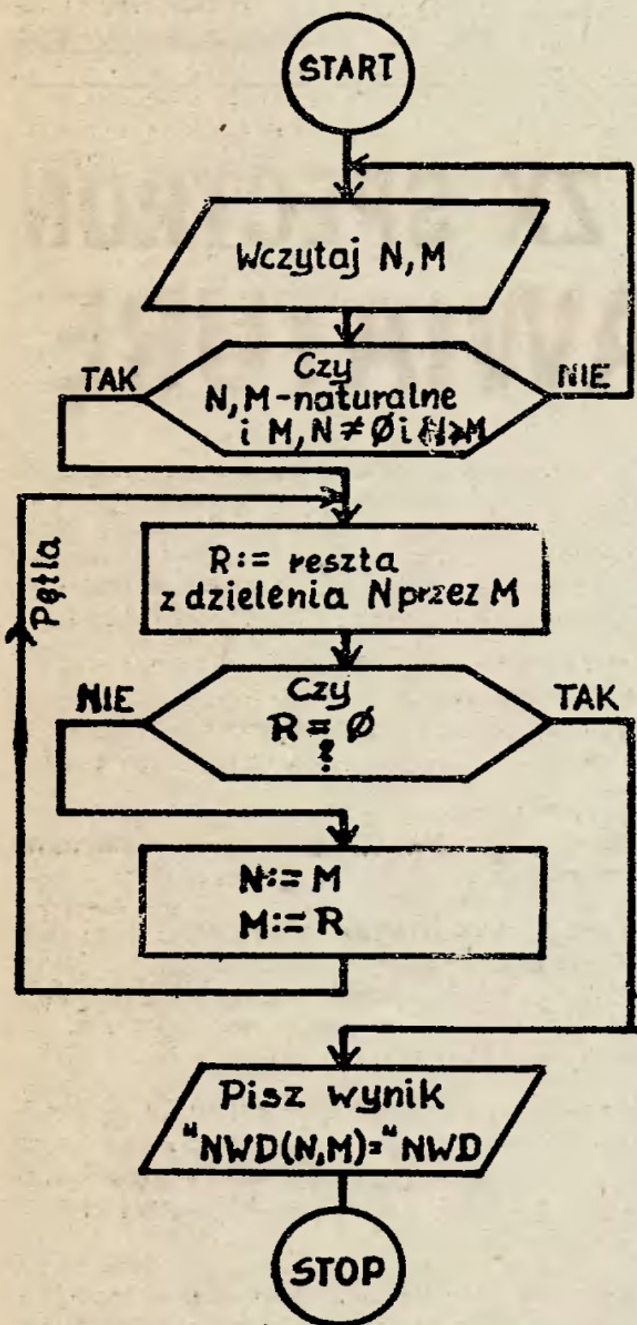
Rys. 3. Schemat blokowy algorytmu Euklidesa.
